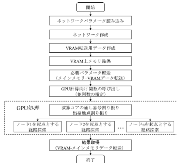
図 1 複数のノードを起点とした経路探索計算の並列化における処理フロー
