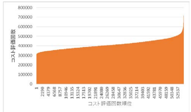
図4 条里制形状ネットワークにおけるコスト評価回数順位
